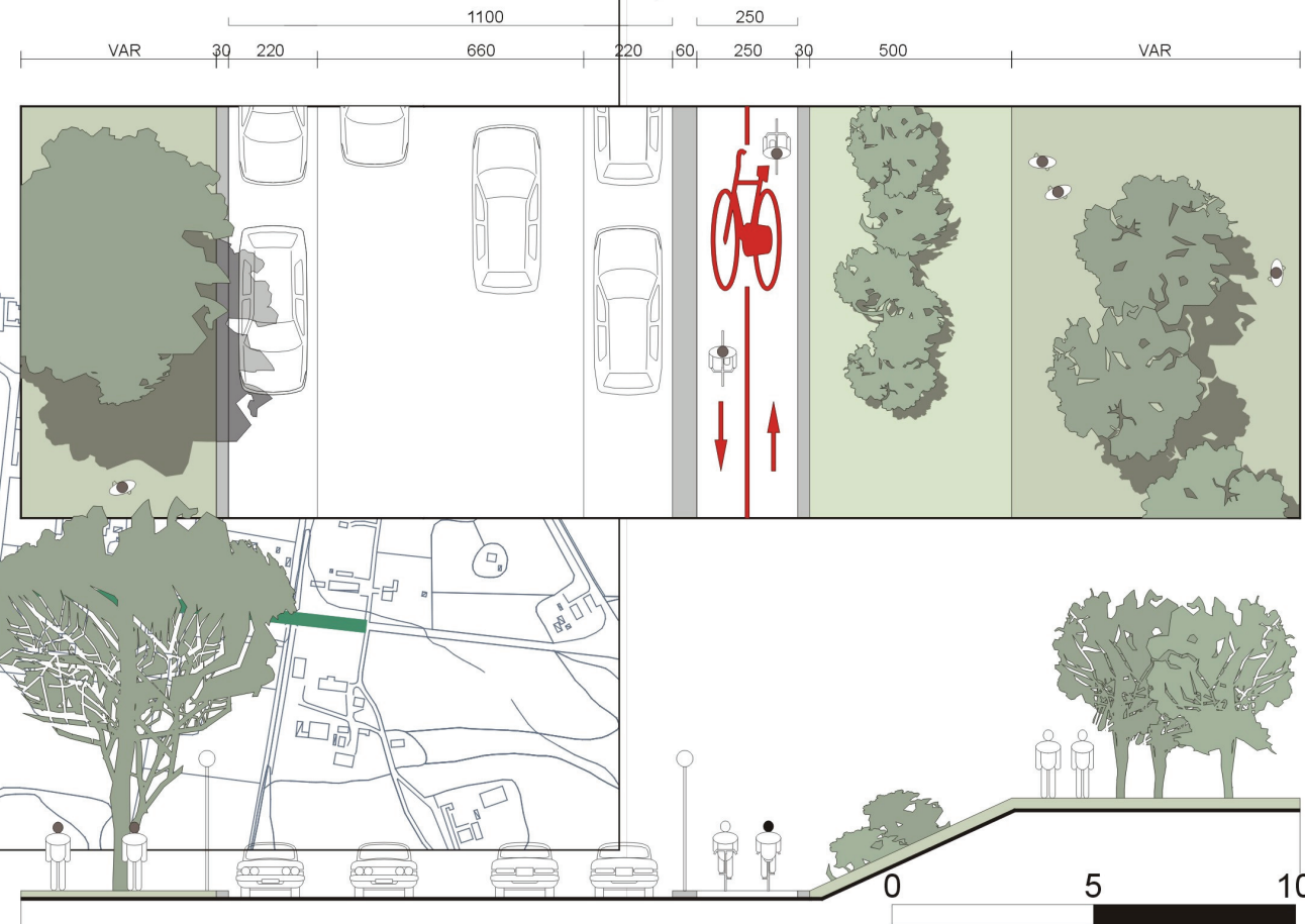
SEZ. Tipo D Circonvallazione - Giardini Comunali
