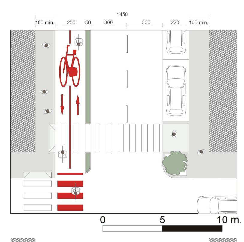
SEZ. Tipo A Via Carlo Alberto
