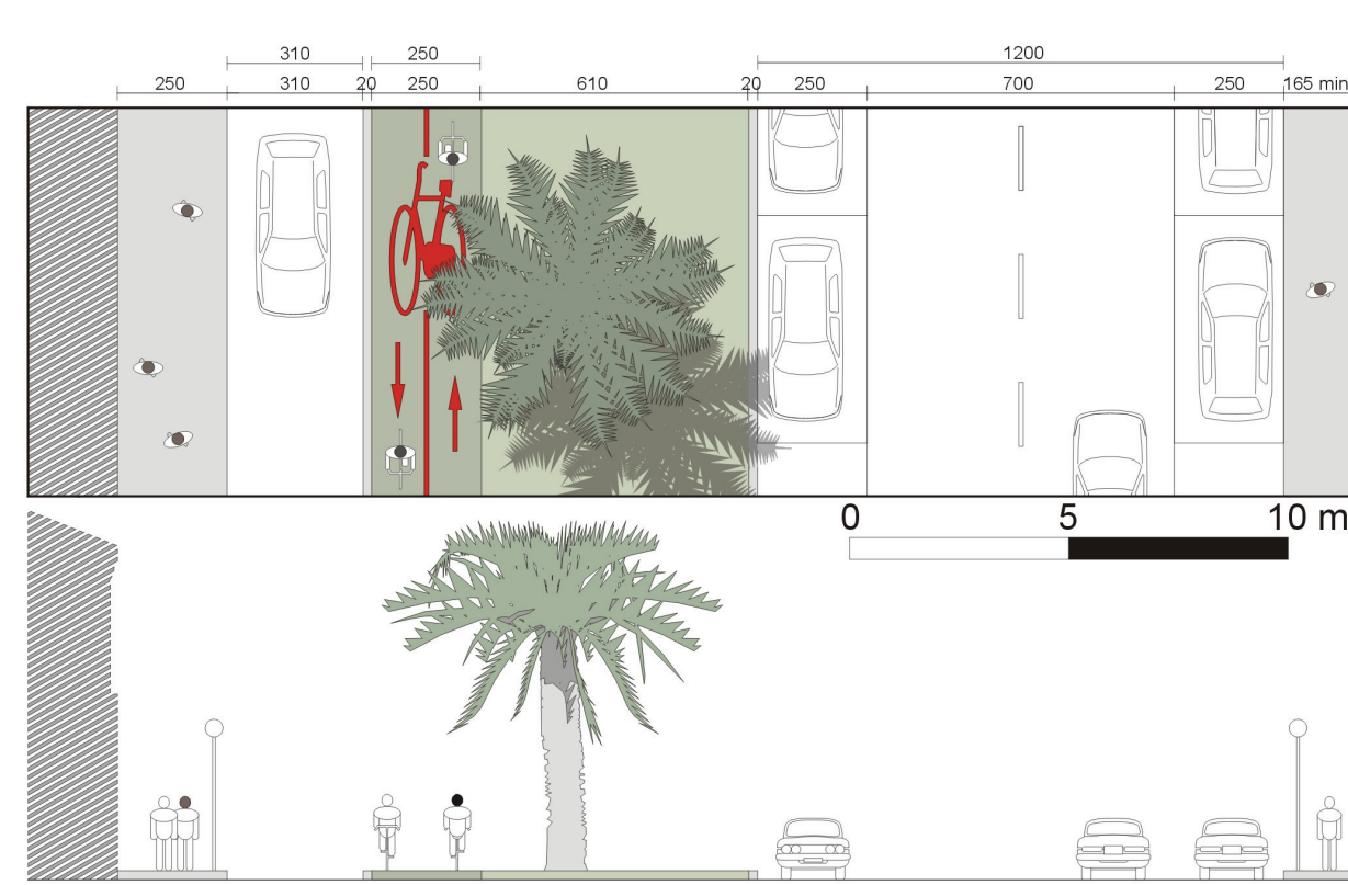
SEZ. Tipo B Via Carlo Alberto
