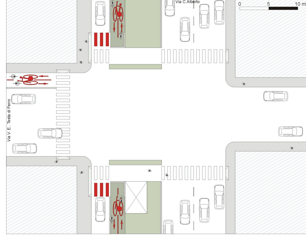
INCROCIO Via Carlo Alberto - Via V. Emanuele Testa di Ferro
