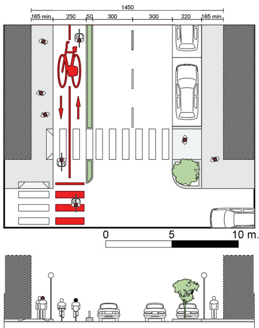
Sezione Tipo
